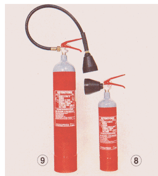
Estintore ad anidride carbonica (CO 2 )
